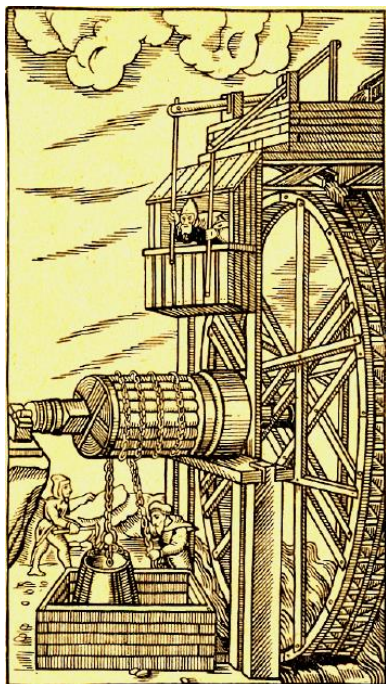
Машина-молот XVв. Вес молота больше тонны
